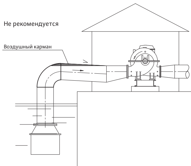
Рис.4. Конструкция всасывающего трубопровода
